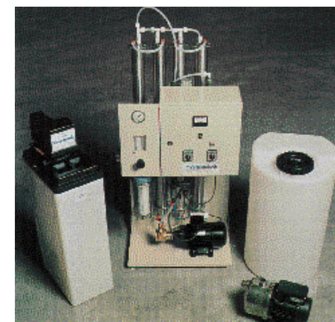
Komplett anläggning med RO-4.2F (kap. 152 liter/timme vid 10 grader råvattentemperatur), avhärtningsfilter som förbehandling, förrådstank och distributionspump.
